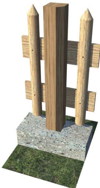
Particolare del punto di incastro del montante al basamento
