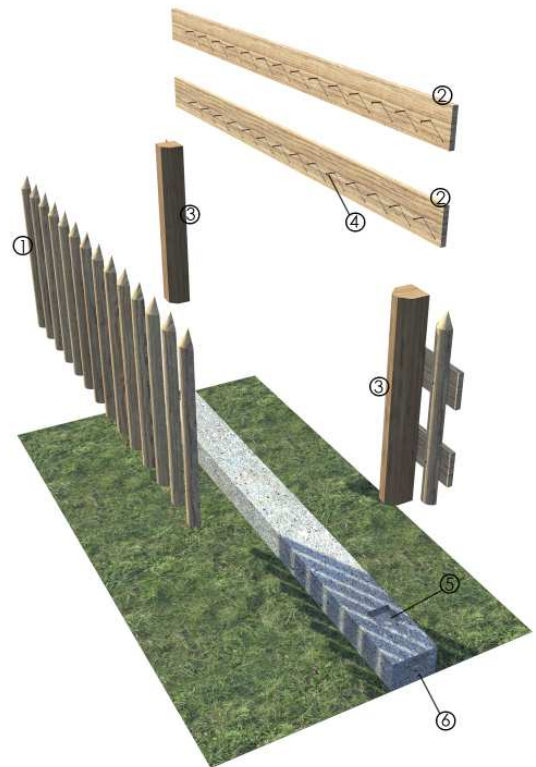
Prospetto della staccionata
