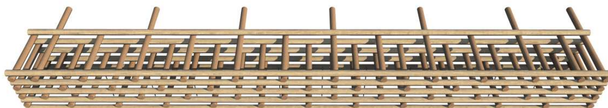
Vista assometrica dello schema di composizione della palificata doppia
