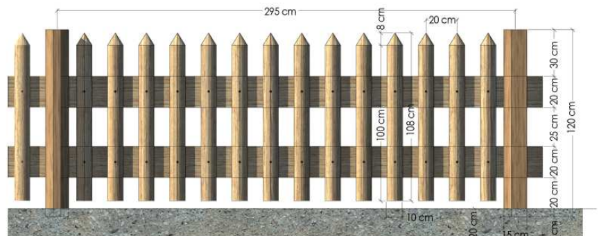
Prospetto della staccionata
